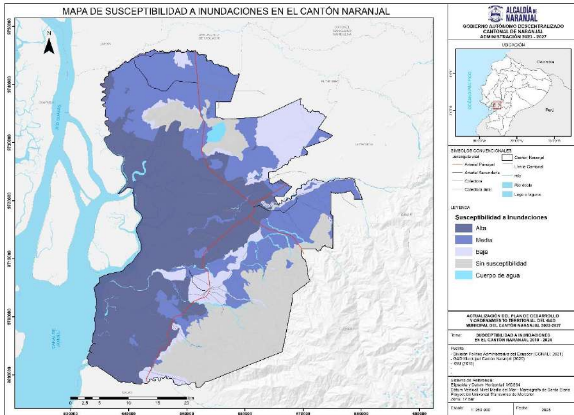
Mapa 76. Susceptibilidad a Inundaciones
