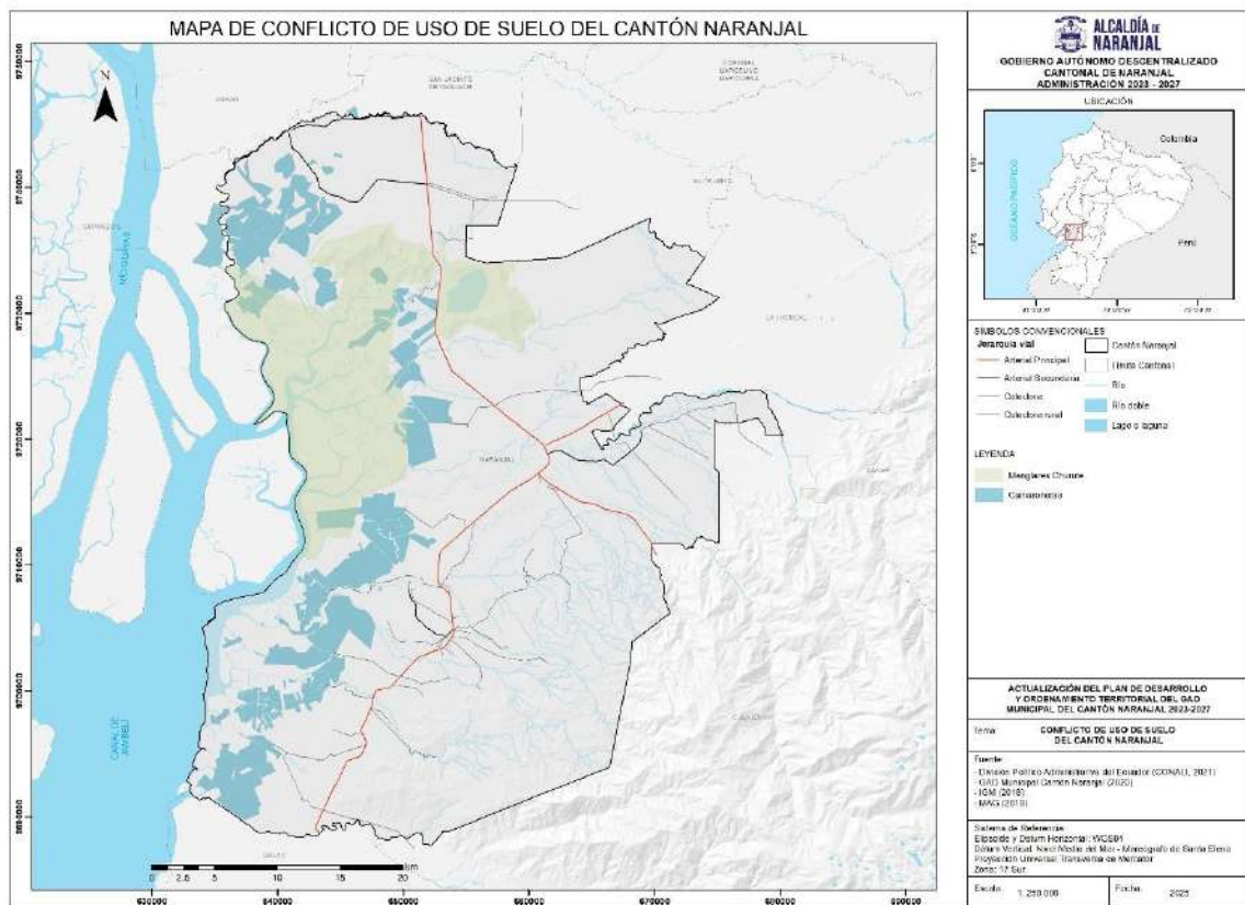
Mapa 20. Conflicto de uso en Naranjal
