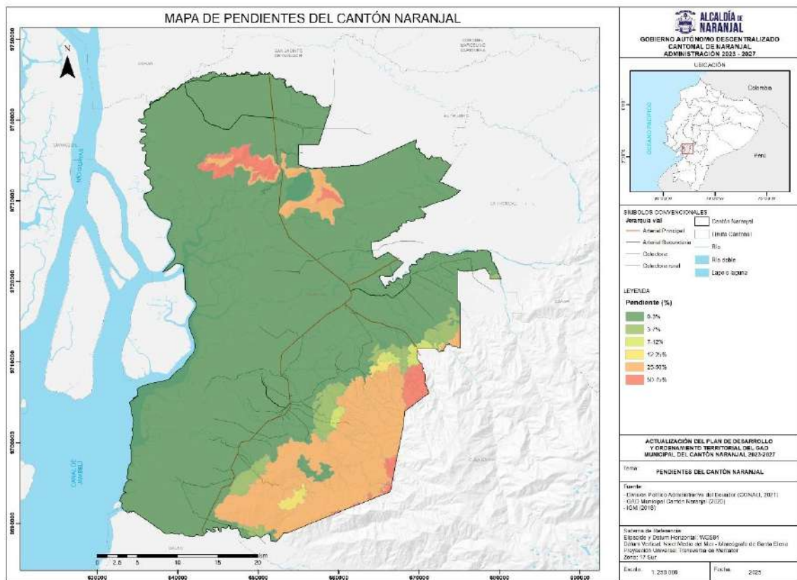
Mapa 3. Pendientes del cantón Naranjal
