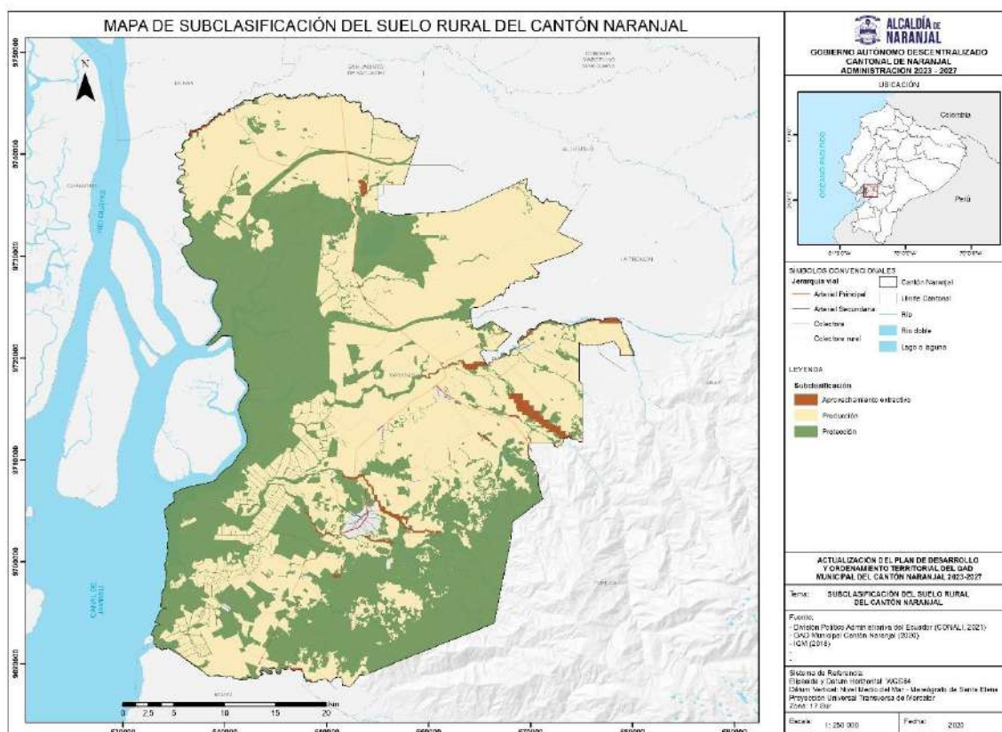
Mapa 35. Subclasificación del suelo Rural del cantón Naranjal
