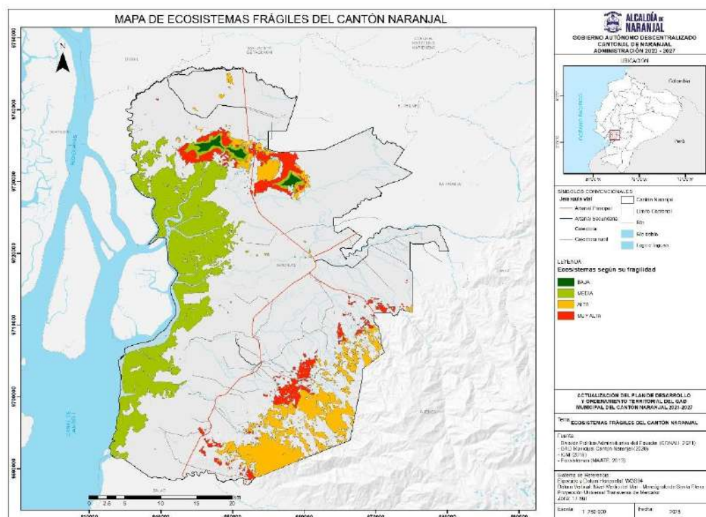
Mapa 13. Ecosistemas según su fragilidad en el cantón Naranjal
