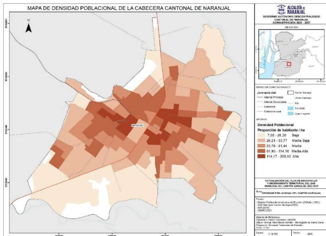
Mapa 27. Densidad Poblacional de la Cabecera Cantonal de Naranjal
